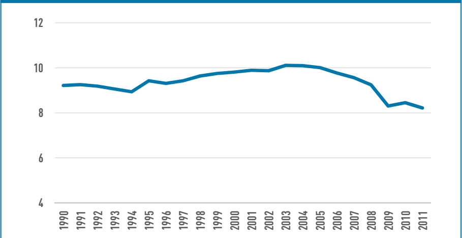
FIGURA 8. Tonnellate di CO 2 equivalente per abitante. Valori concatenati anno di riferimento 2005. Anni 1990-2011
